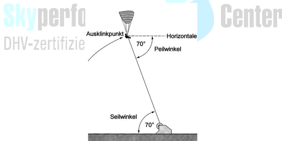
Abbildung 14 Ausklinkhöhe
