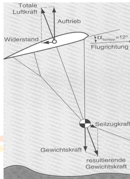
Abbildung 12 Kräfteverteilung beim Windschlepp
