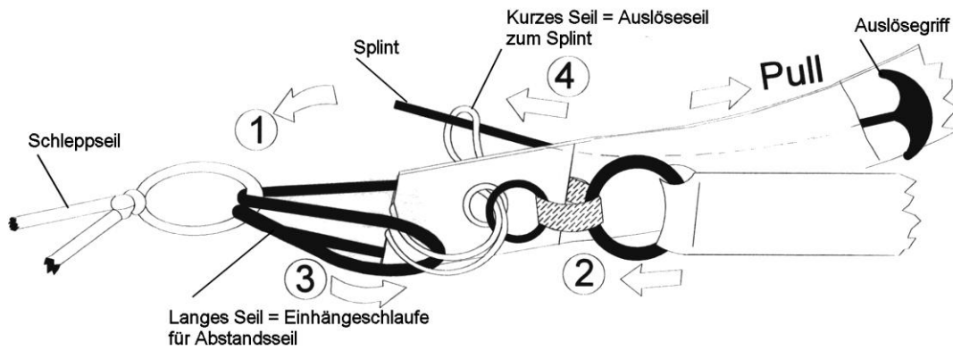
Abbildung 9 Einhängemechanismus Klinke – Schleppeil
