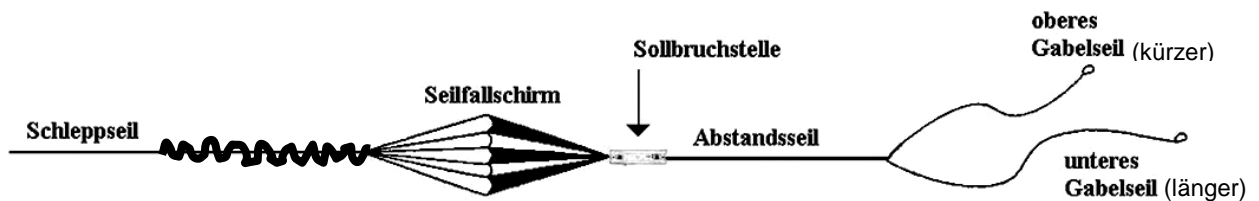
Abbildung 5 Vorseil
