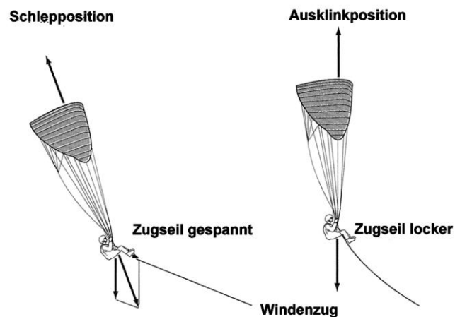
Abbildung 16 Schleppseil straff und locker
