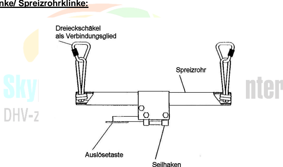
Abbildung 7 Spreizrohrklinke
