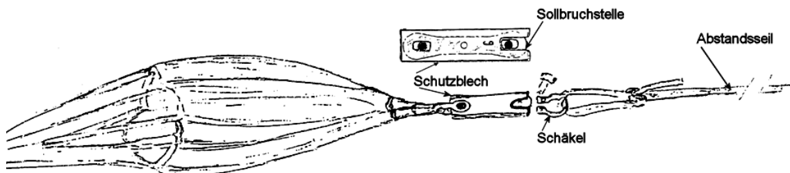
Abbildung 6 Sollbruchstelle
